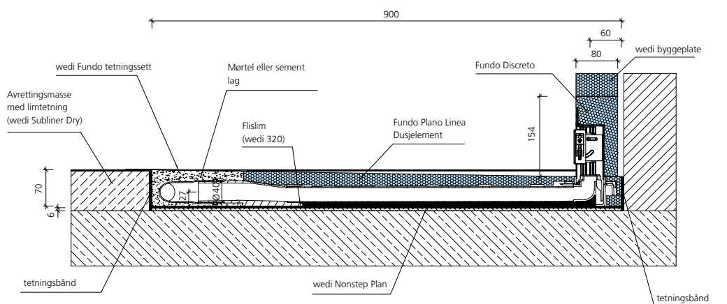
Fundo Discreto, veggavløp, DN 40, avrettingsgulv
