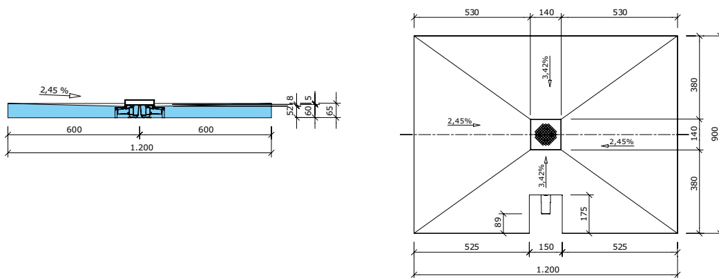
Fundo Plano, komplett system B, tilkobling på kortsiden
