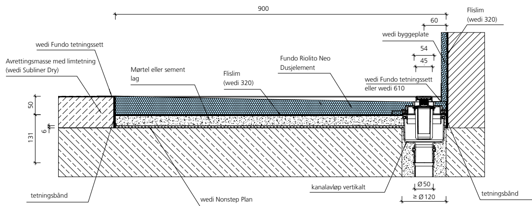
wedi Fundo kanalavløp vertikalt, DN 50, avrettingsgulv
