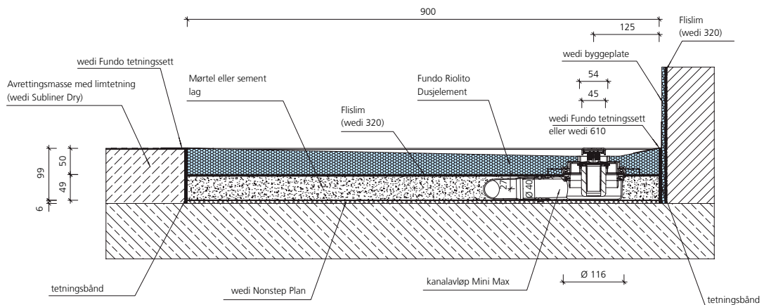
wedi Fundo kanalavløp Mini Max, DN 40, avrettingsgulv
