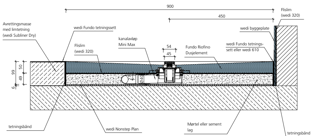
wedi Fundo kanalavløp Mini Max, DN 40, avrettingsgulv
