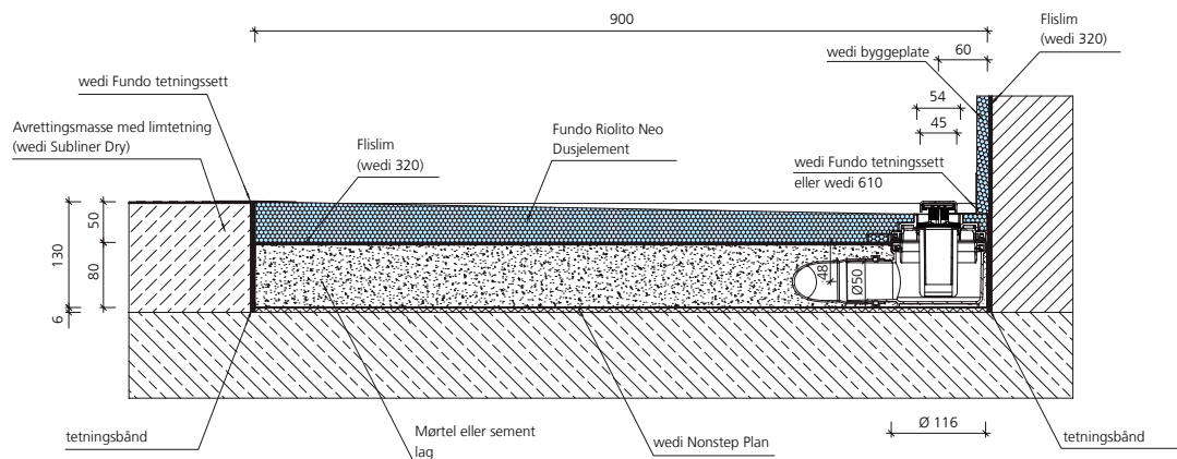
wedi Fundo kanalavløp horisontalt, DN 50, avrettingsgulv
