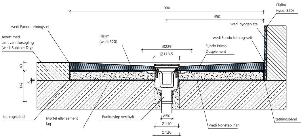
wedi Fundo punktavløp vertikalt, DN 50, avrettingsgulv
