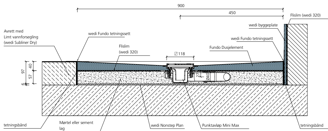
wedi Fundo punktavløp Mini Max, DN 40, avrettingsgulv
