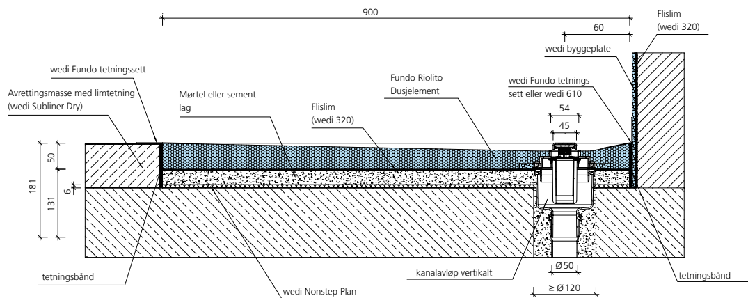
wedi Fundo kanalavløp vertikalt, DN 50, avrettingsgulv
