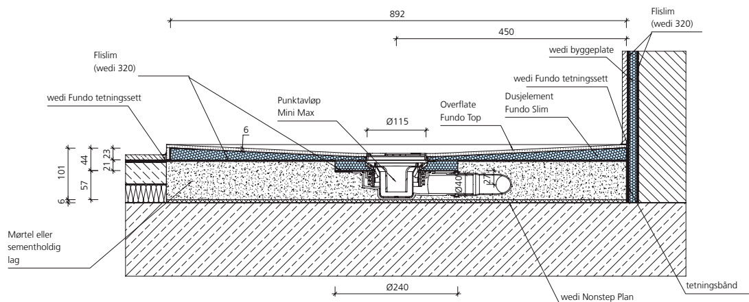
wedi Fundo punktavløp Mini Max, DN 40, på avrettingsgulv
