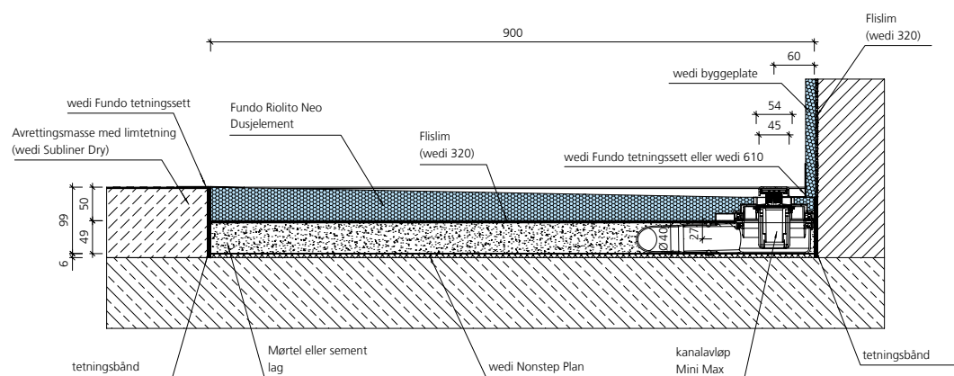
wedi Fundo kanalavløp Mini Max, DN 40, avrettingsgulv
