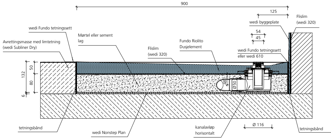
wedi Fundo kanalavløp horisontalt, DN 50, avrettingsgulv
