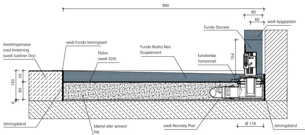
Fundo Discreto, veggavløp, DN 50, avrettingsgulv
