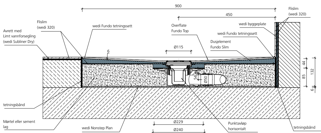
wedi Fundo horisontalt punktavløp, DN 50, i avrettingsgulv
