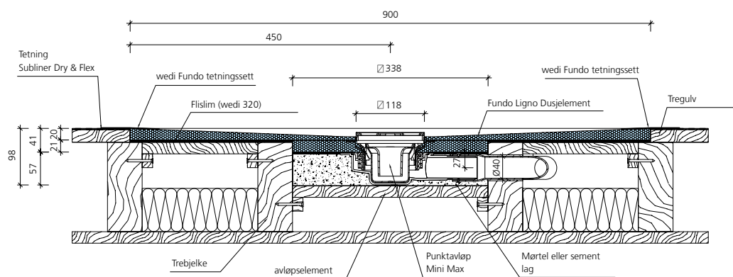
wedi Fundo punktavløp Mini Max, DN 40, i bjelkelag
