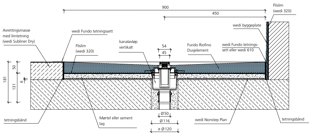
wedi Fundo kanalavløp vertikalt, DN 50, avrettingsgulv
