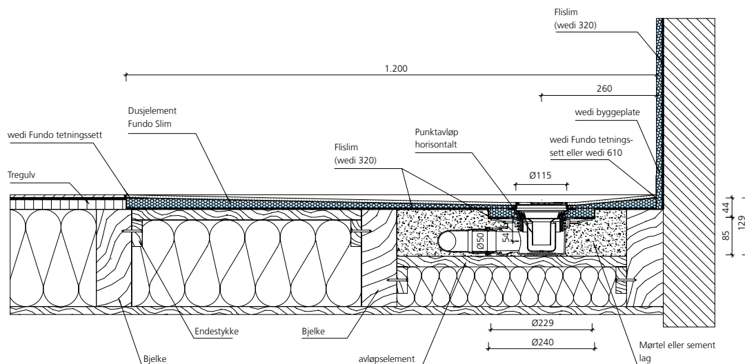
wedi Fundo horisontalt punktavløp, DN 50, i trebjelkeunderlag
