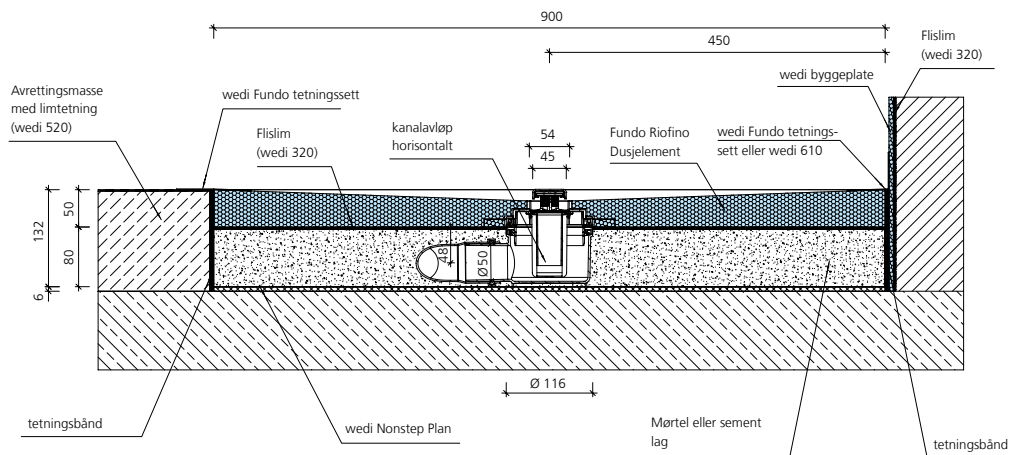
wedi Fundo kanalavløp horisontalt, DN 50, avrettingsgulv
