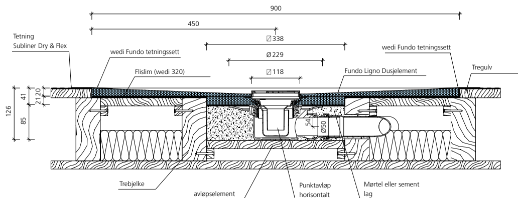
wedi Fundo horisontalt punktavløp, DN 50, i bjelkelag
