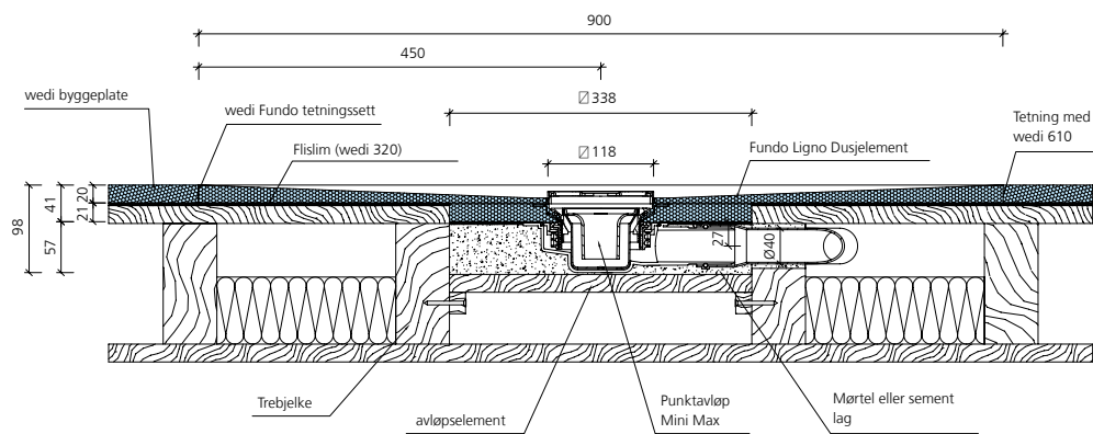
wedi Fundo punktavløp Mini Max, DN 40, på bjelkelag
