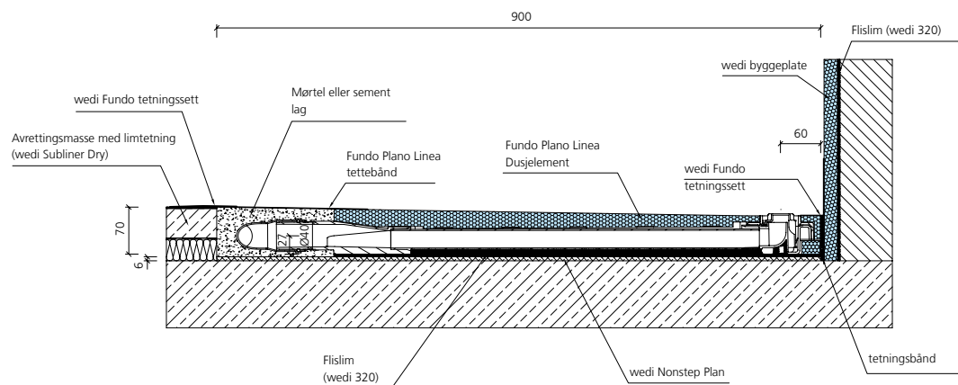
Fundo Plano Linea, integrert horisontalt avløp, DN 40, avrettingsgulv
