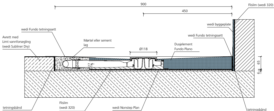
Fundo Plano, integrert horisontalt avløp, DN 40, avrettingsgulv
