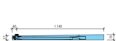
Fundo Plano Linea, dusjelement med kort kanal
