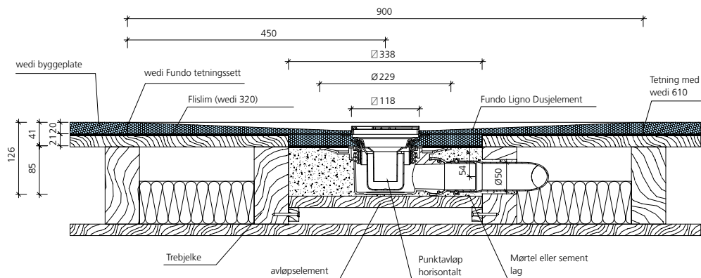
wedi Fundo horisontalt punktavløp, DN 50, på bjelkelag
