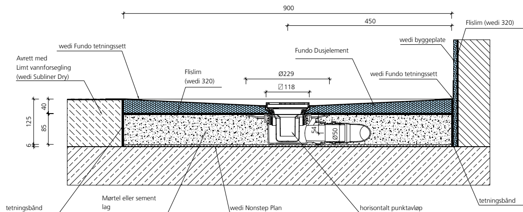
wedi Fundo horisontalt punktavløp, DN 50, avrettingsgulv
